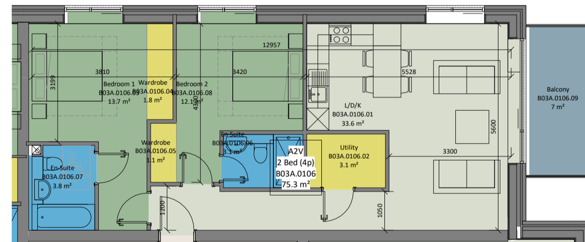
⑥ Unit Type A2V 1:100
