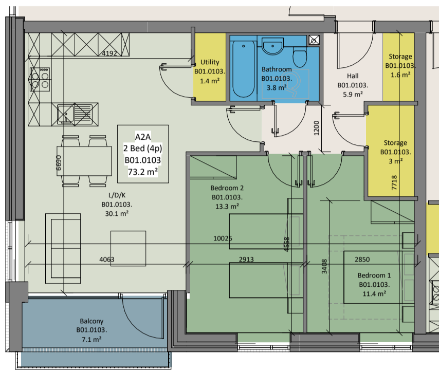
① Unit Type A2A 1:100
