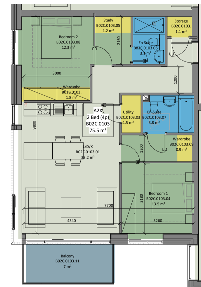
⑧ Unit Type A2X 1:100
