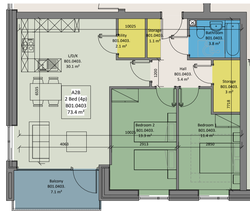
⑬ Unit Type A2B 1:100
